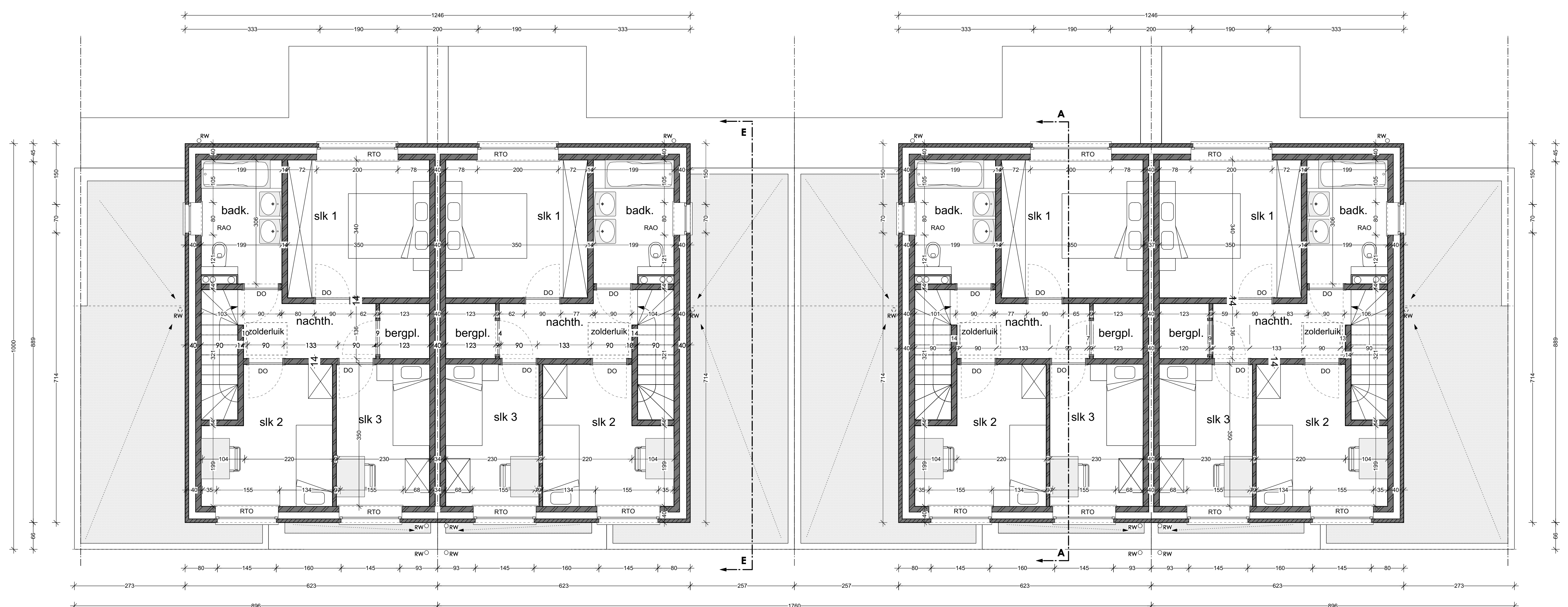
BOUWBLOK A, VERDIEPINGSPLAN
