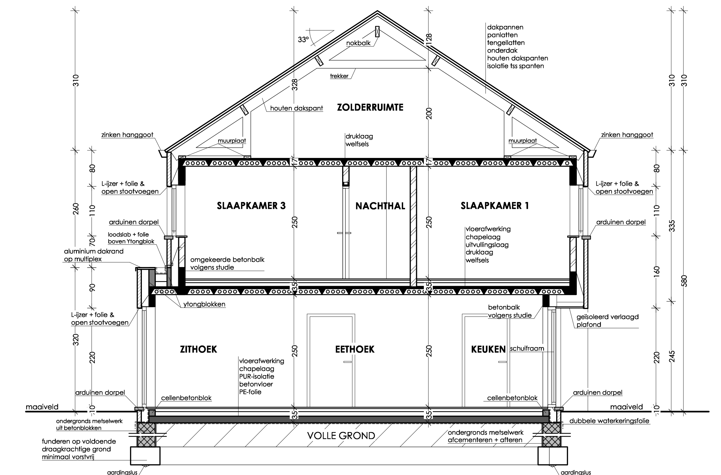
DOORSNEDE AA: BLOK A
