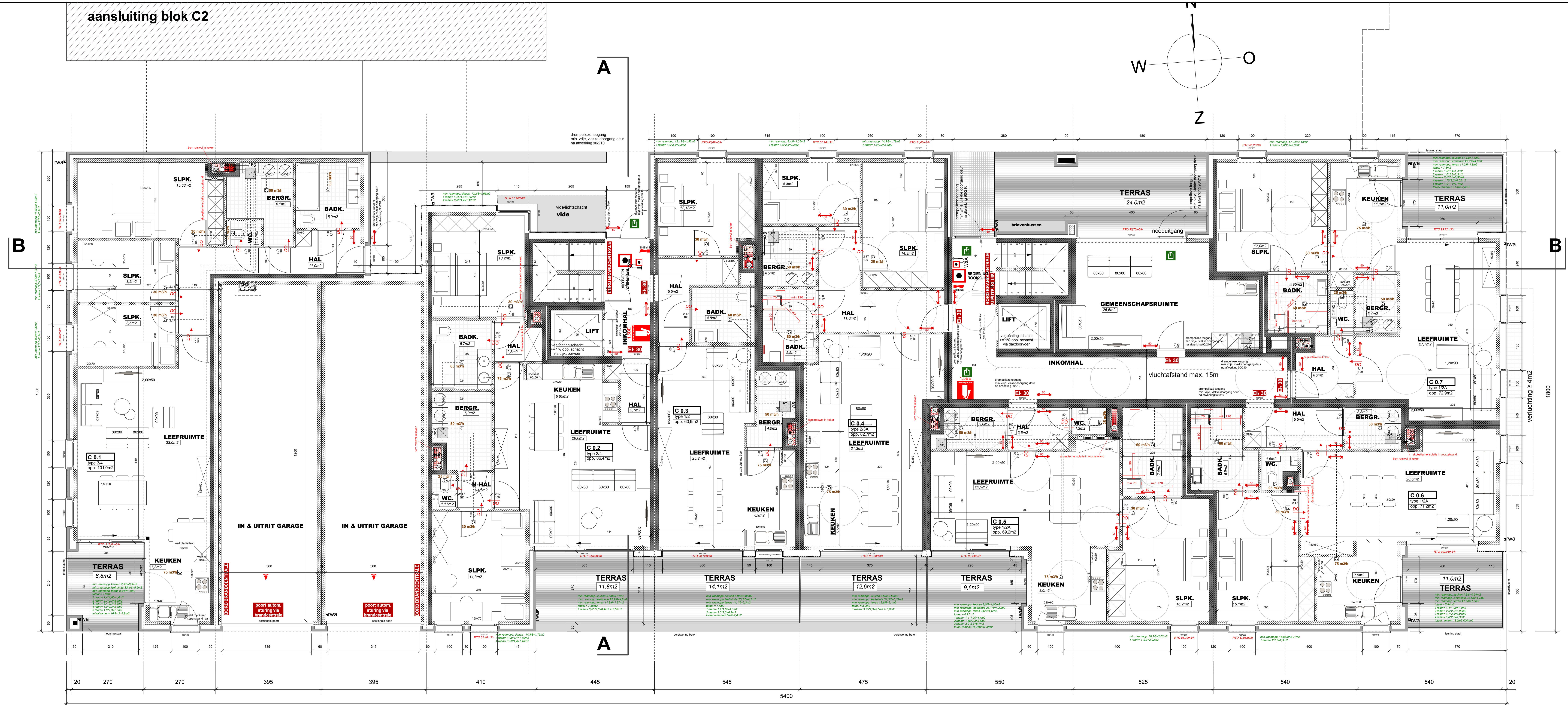
GELIJKVLOERS 0 BLOK C1 SCHAAL 1:50
